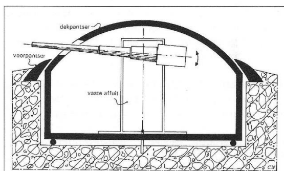
afb.46 Principe van een pantserkoepel
