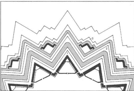
e. Getenaillerd stelsel.
