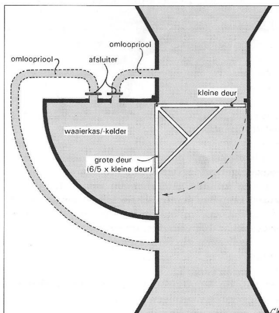
afb.72 Waaiersluis (schematische weergave)
