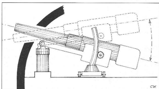
afb.41 Minimaalschietgataffuit
