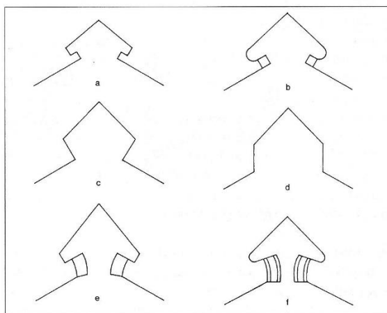
afb.7 Basisvormen van bastions.
