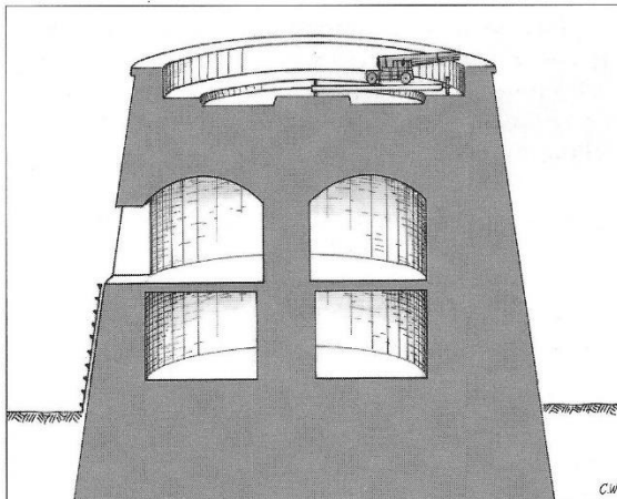
afb.38 Martellotoren (doorsnede)
