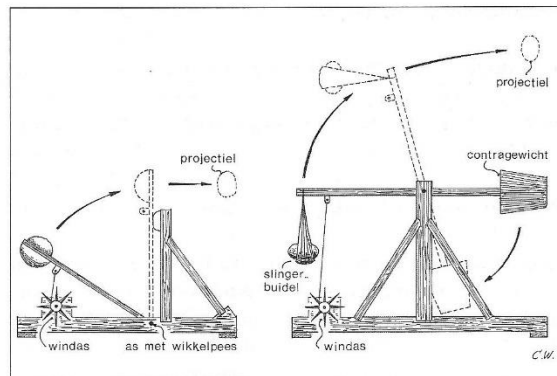
afb.11 Lepelblijde (links) en slingerblijde (rechts)
