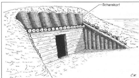
afb.10 Blinding, met toepassing van schanskorven
