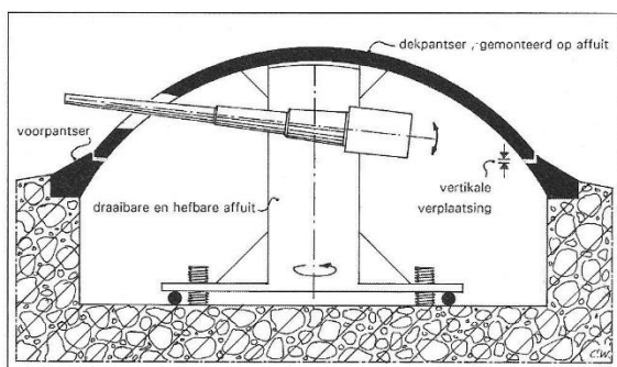
afb.44 Principe van een pantseraffuit
