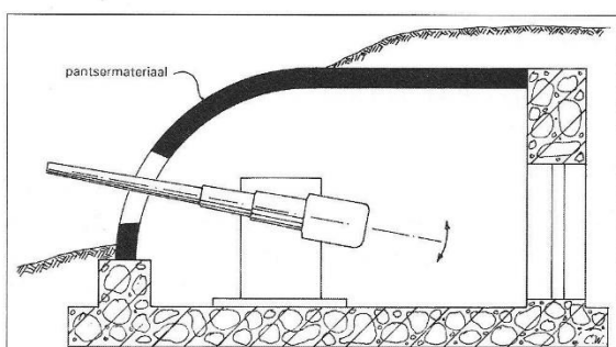
afb.45 Principe van een pantserkazemat
