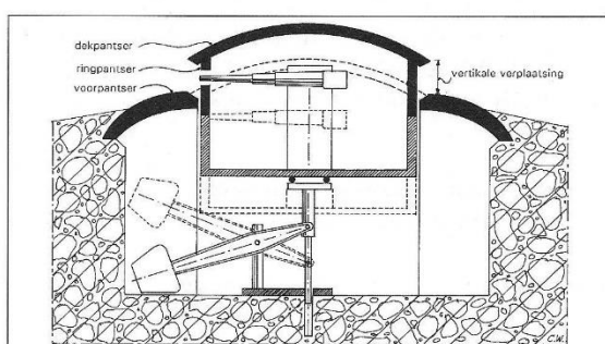
afb.47 Principe van een hefkoepel
