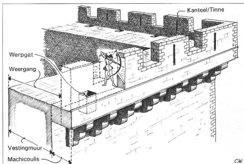
afb.73 Weergang, kantelen en machicoulis op een vestingmuur
