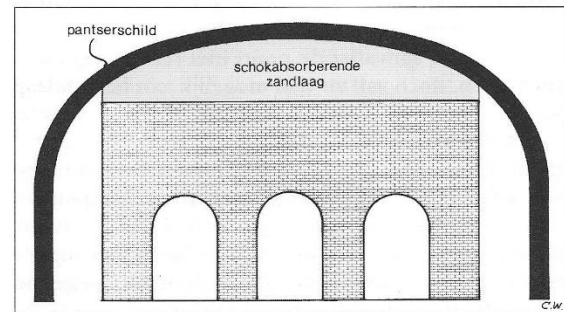
afb.14 Principe van een carapace (doorsnede)
