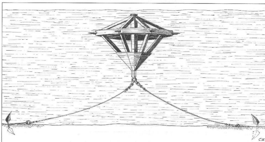
afb.36 Kunstklip
