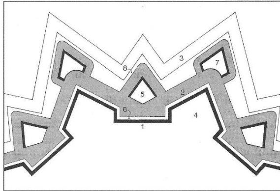
b. Oud-Nederlands stelsel.
