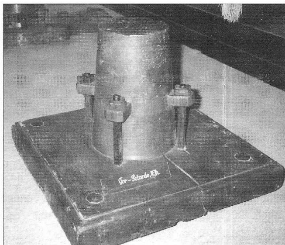
afb.48 Pétard(e) (foto: P.C. van Kerkum)
