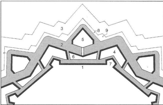
c. Frans stelsel (Vauban's 2 e methode).
