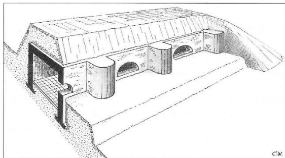
afb.51 Reiche-kazemat
