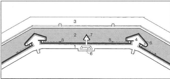
a. Oud-Italiaans stelsel.
