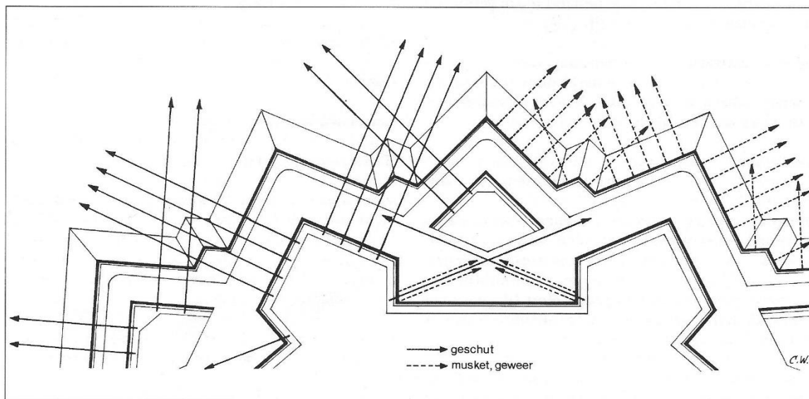
afb.30 Hoofdschootsrichtingen (vanaf een gebastioneerd verdedigingswerk)
