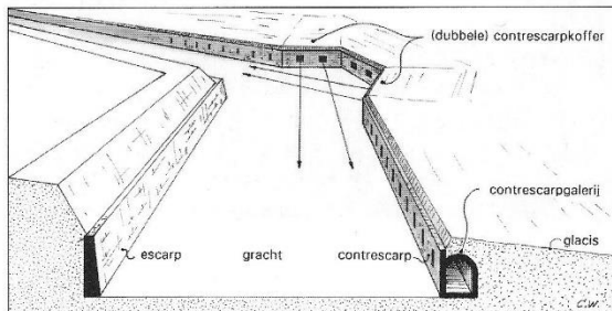
afb.19 Contrescarpgalerij (betekenis 1) met dubbelecontrescarpkoffer
