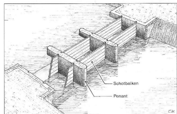
afb.56 Schotbalksluis (dubbel) met tussengelegde penanten
