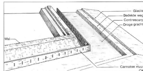
afb.15 Carnotse muur
