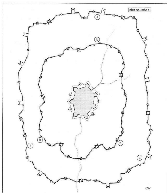
afb.16 Circumvallatielinie (a) en contravallatielinie (b) rond een belegerde vesting
