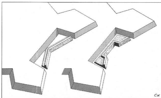
afb.62 Tenailles (grondvormen, betekenis 1)
