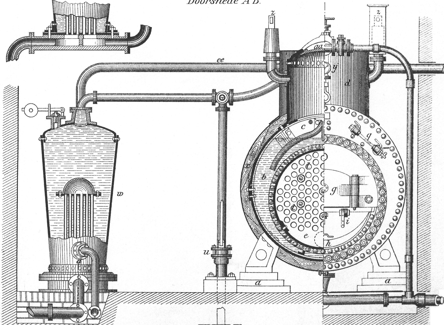
Tekening stoomketel met voorwarmer
